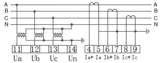
三相四线电压电流互感器接入
