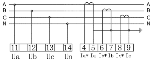
三相四线电流互感器接入
