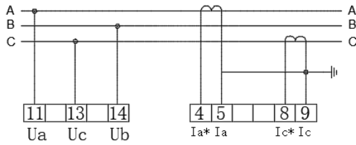
三相三线电流互感器直接接入
