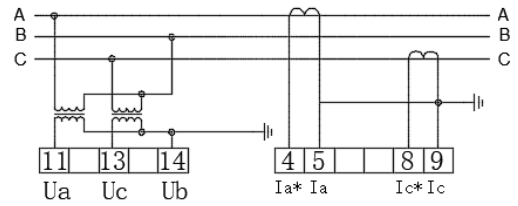
三相三线电压电流互感器接入
